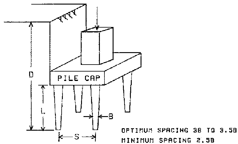
a. PILES
