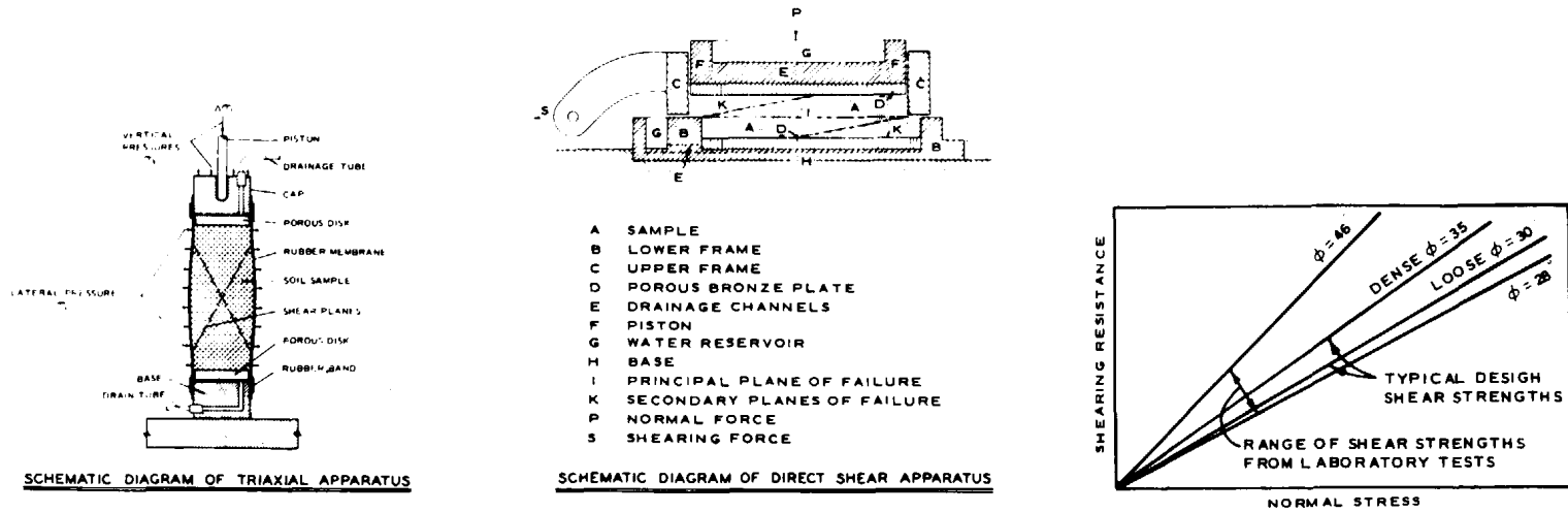
a. SHEAR TEST APPARATUS
